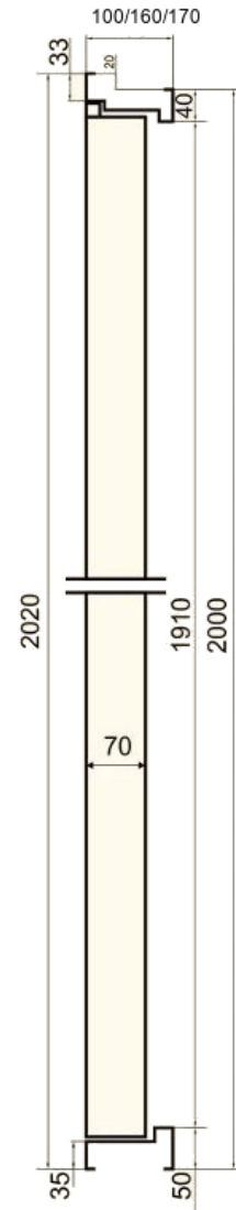
Zvislý rez
